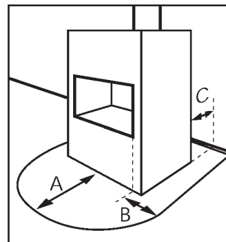
fig. 1: Dimensions de la plaque au sol
