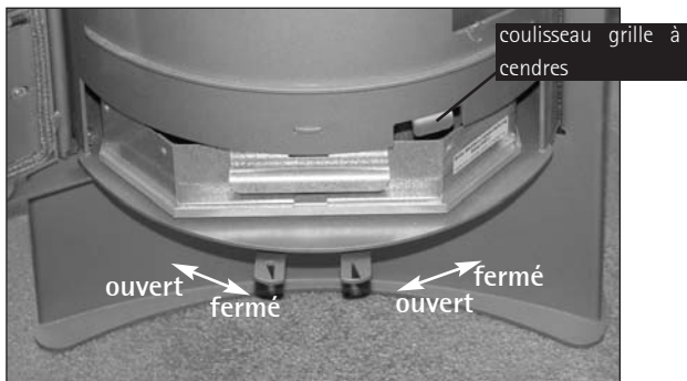
curseur de ventilation primaire (I)
