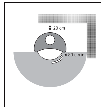
fig. 2: Zone de rayonnement de la porte vitrée du poêle
